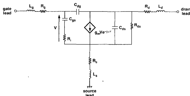
Fig. 2. A FET equivalent circuit.
